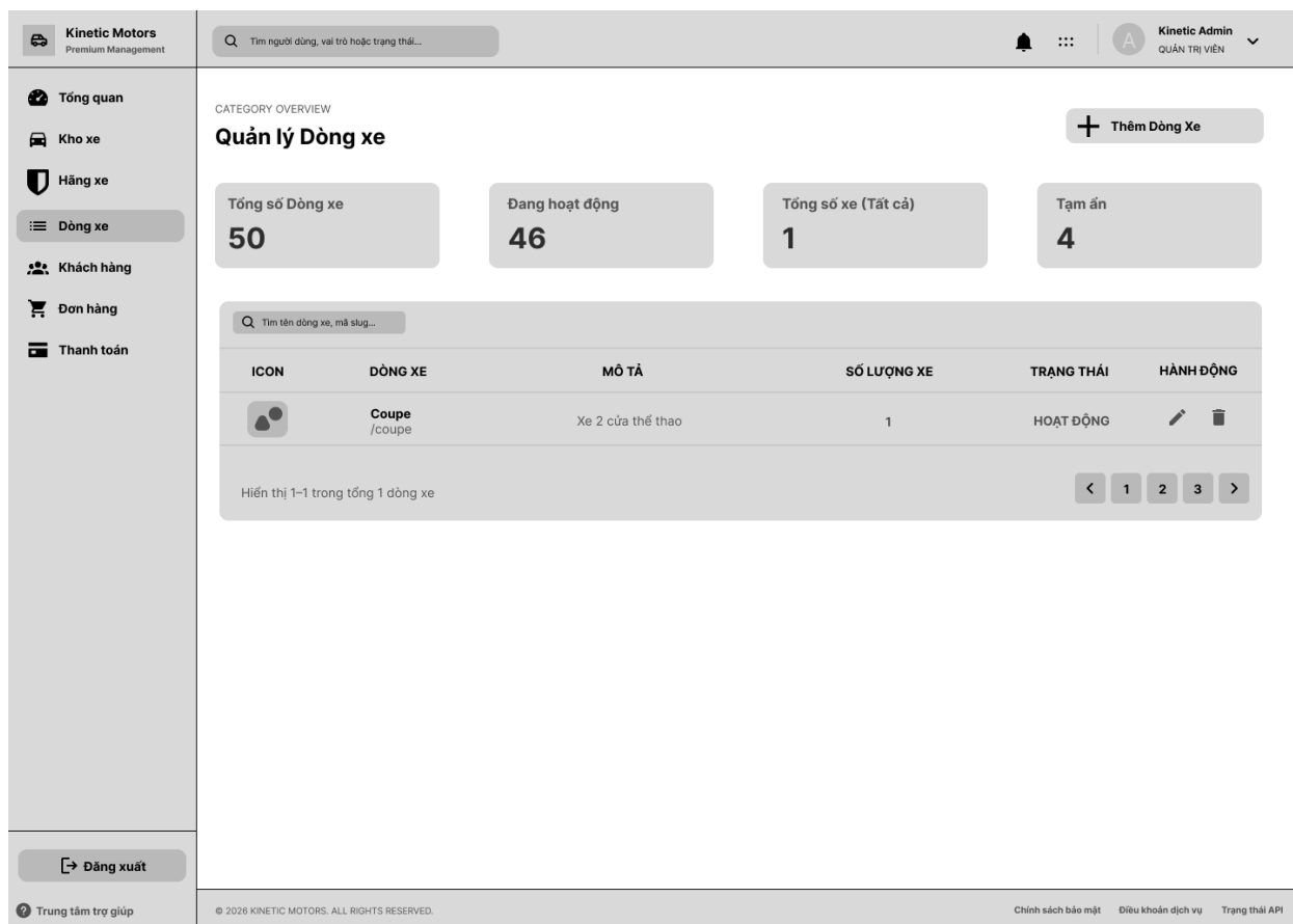
Hình 2.9 Wireframe trang quản lý dòng xe
