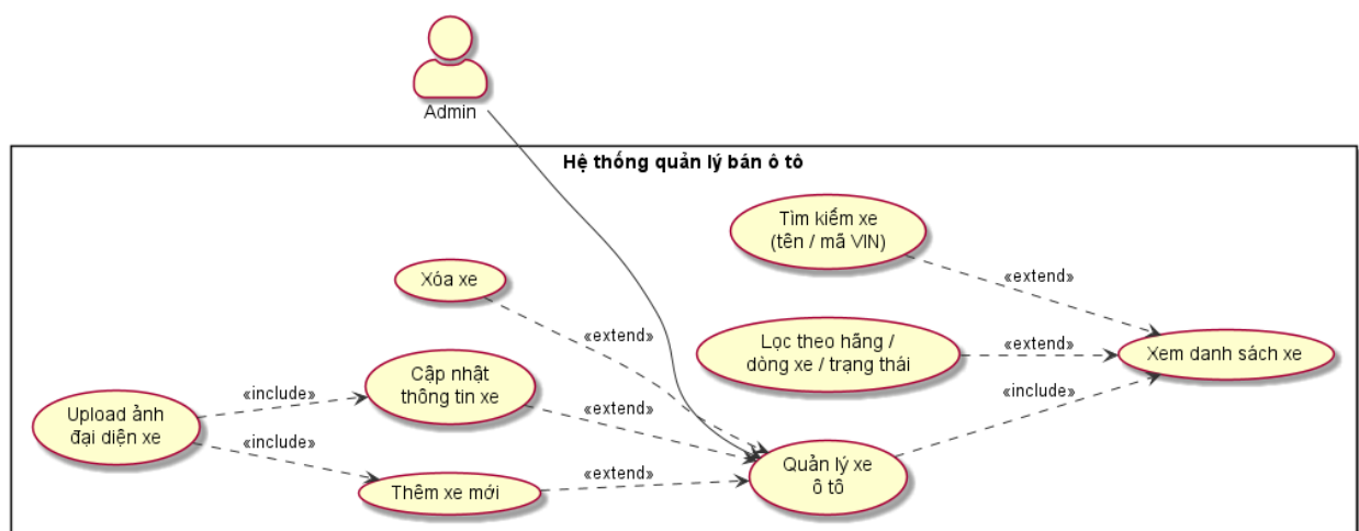
Hình 1.4 Use Case quản lý xe
