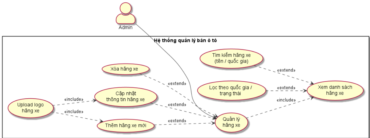
Hình 1.5 Use Case quản lý hãng xe
