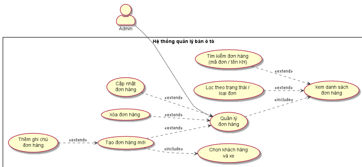
Hình 1.8 Use Case quản lý đơn hàng
