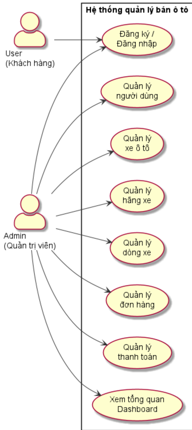
Hình 1.1 Use Case tổng quát
