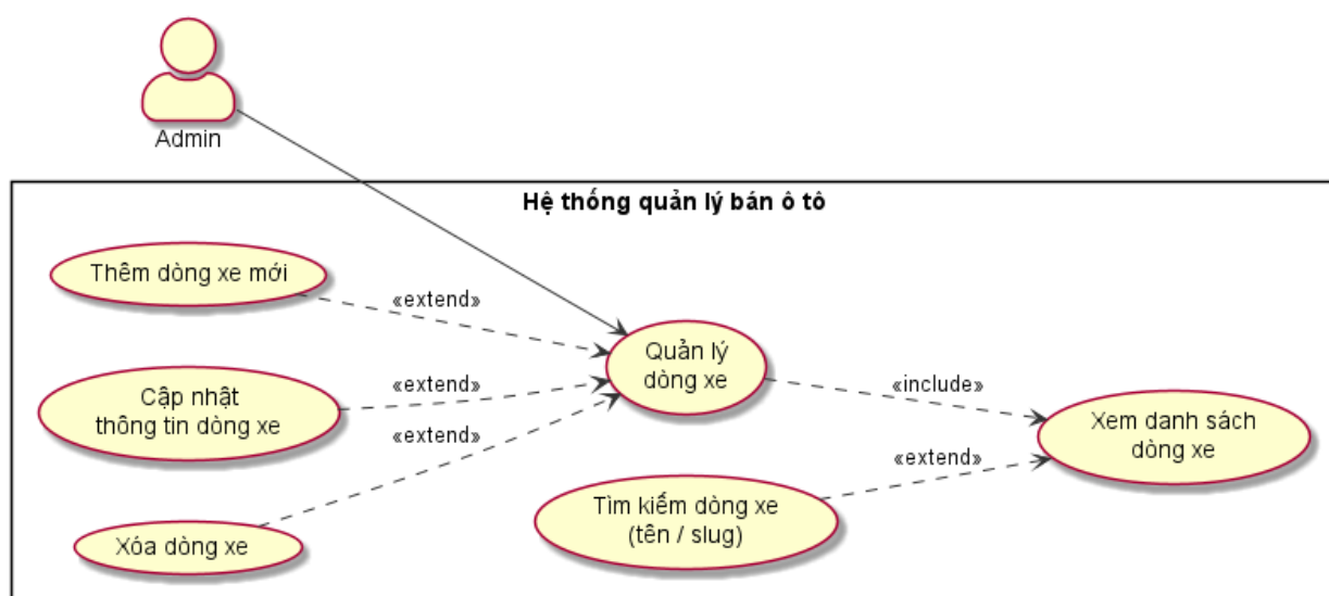
Hình 1.6 Use Case quản lý dòng xe
